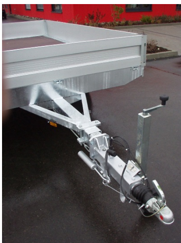
Ausziehbare Deichsel mit selbst- einstellendem Bremsgestänge
