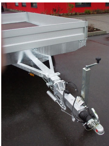
Ausziehbare Deichsel mit selbst- einstellendem Bremsgestänge
